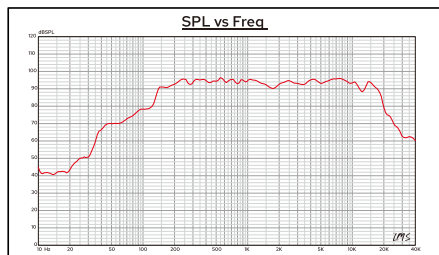
频响曲线
